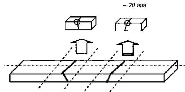
Fig. 2.6.8.3.1.1.1 Sectioning plan
