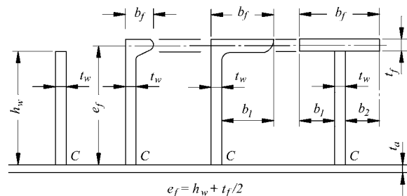
Fig. 7.10.6.31 Dimensions of stiffener
