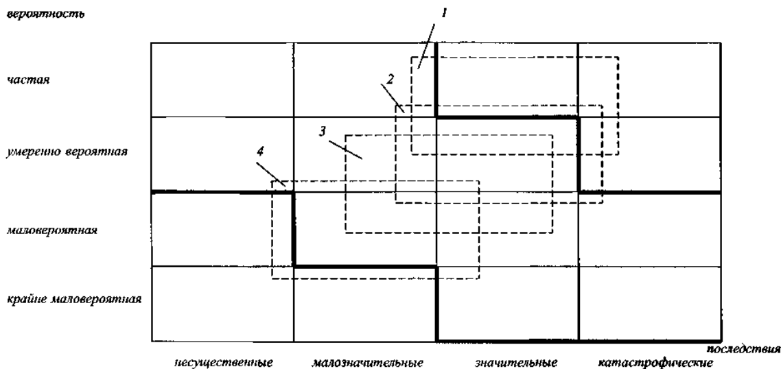
Рис. 2.2.2.4.2 Качественная матрица рисков при пожарах:
