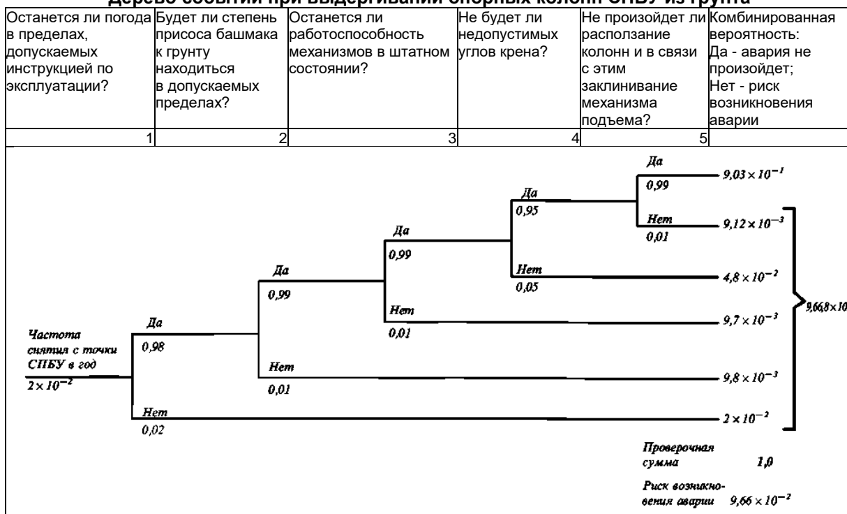
Дерево событий при выдергивании опорных колонн СПБУ из грунта
