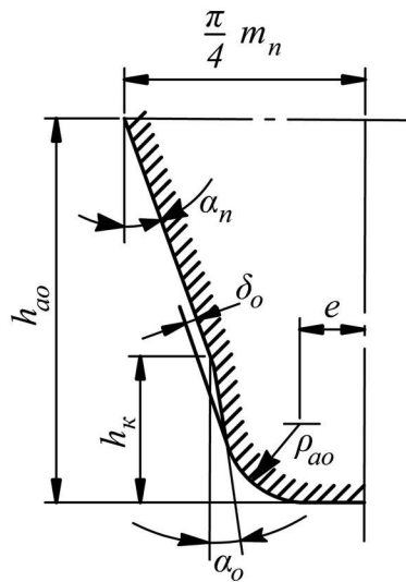
Fig. 4.2.2.7.3.2-3 Protuberance hob
