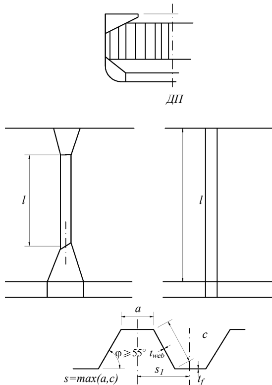
Рис. 2.3: n — нейтральная ось гофра; l f — толщина нетто пояса гофра; t web — толщина стенки гофра
