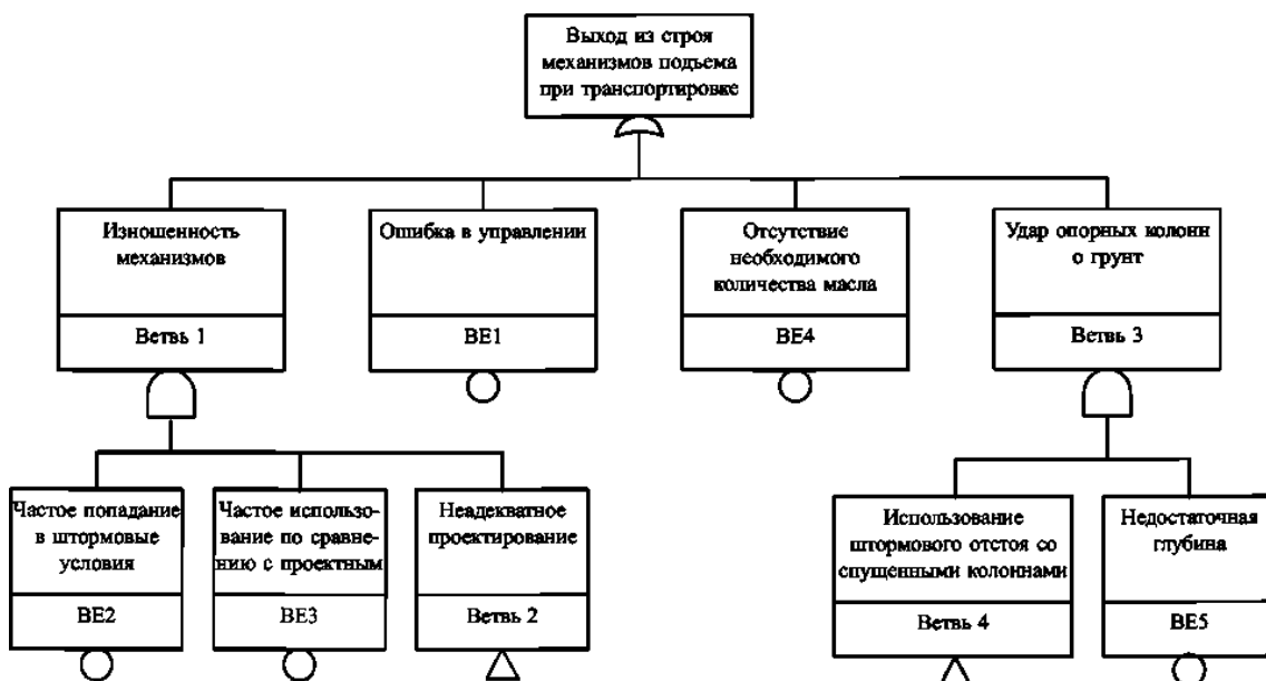
Начальное построение дерева ошибок и неполадок
