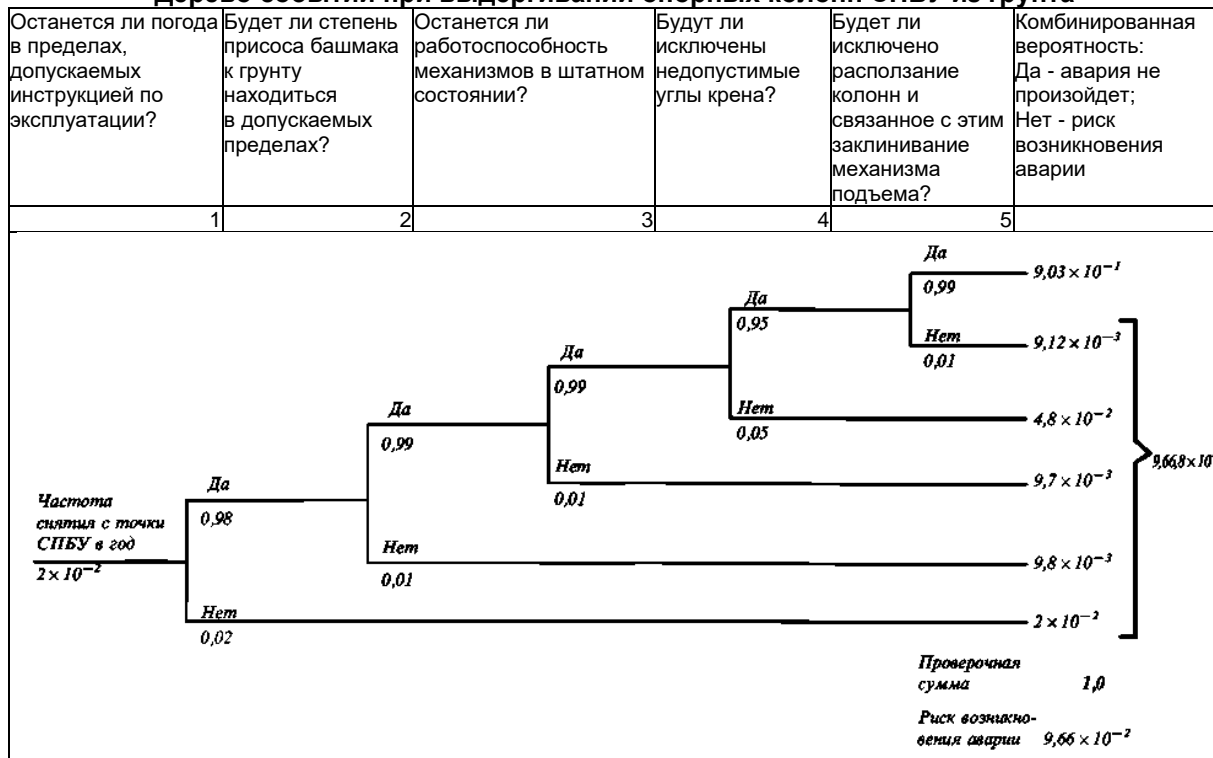
Дерево событий при выдергивании опорных колонн СПБУ из грунта
