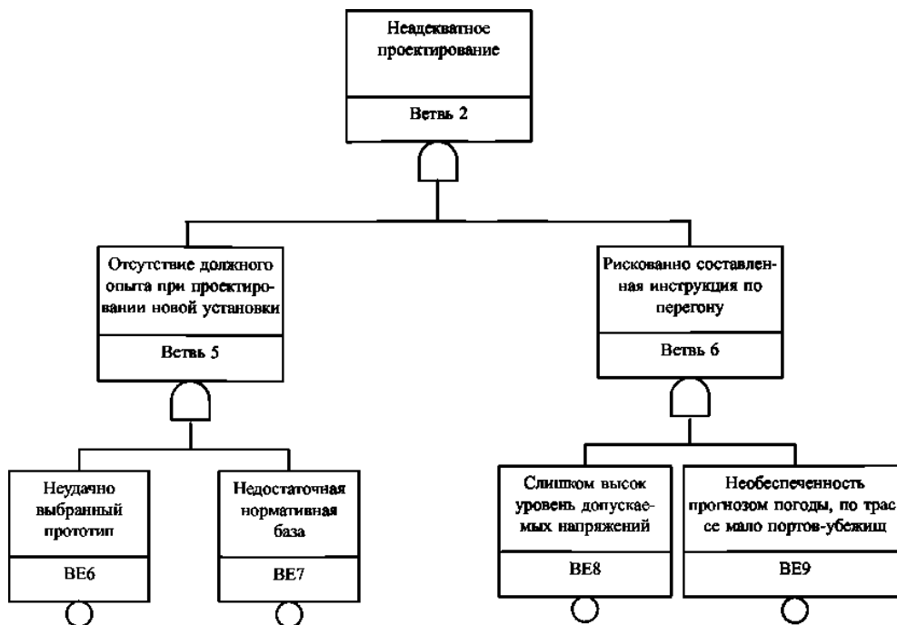
Продолжение построения дерева ошибок и неполадок
