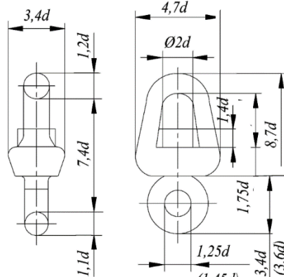
Fig. 7.1.3-7 Swivel
