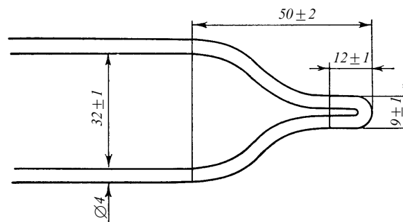
Fig. 1 Filament loop
