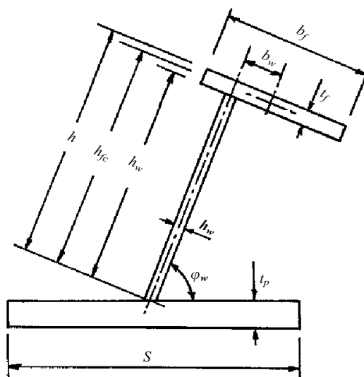
Рис. 1.2.5.7 Геометрия ребра жесткости
