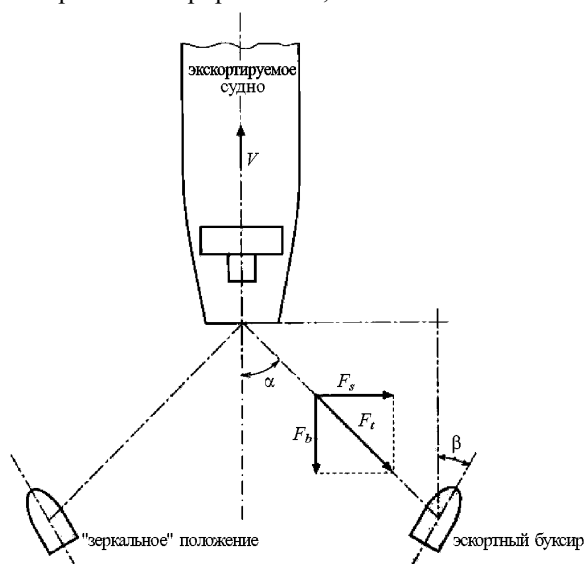
Рис. 2.1.2.1 Типовая схема эскортных операций
