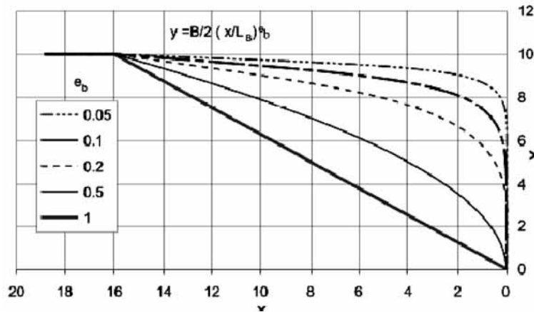
Рис. 1.2.13.2.1-1 Определение формы носовой оконечности
