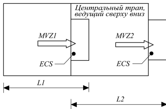
Рис. 2.2.1.2-1 Эвакуационный трап обслуживает одну главную вертикальную зону
