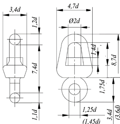
Fig. 7.1.3-7 Swivel
