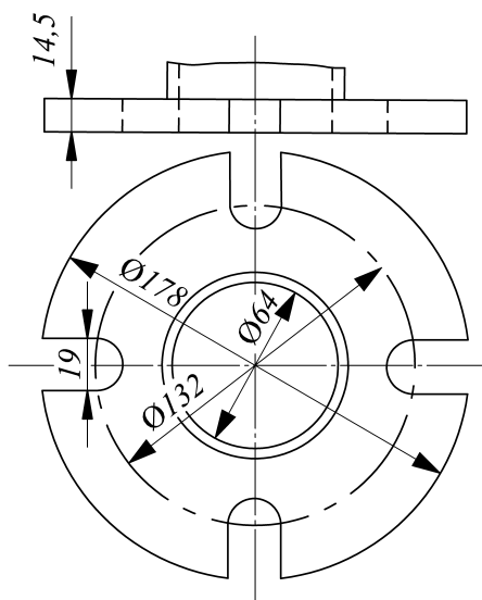
Рис. 5.1.18 Международное береговое соединение (судно)
