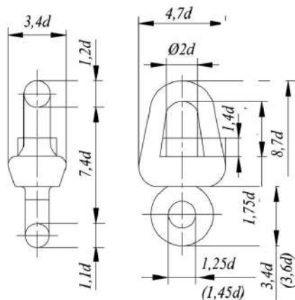
Fig. 7.1.3-7 Swivel
