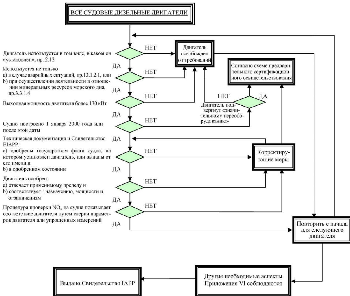
Рис. 2 Первоначальное освидетельствование на судне
