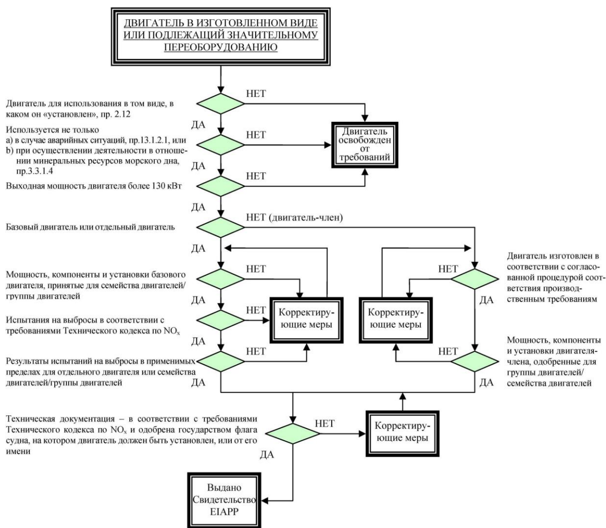
Рис. 1 Освидетельствование на стенде предприятия (изготовителя)
