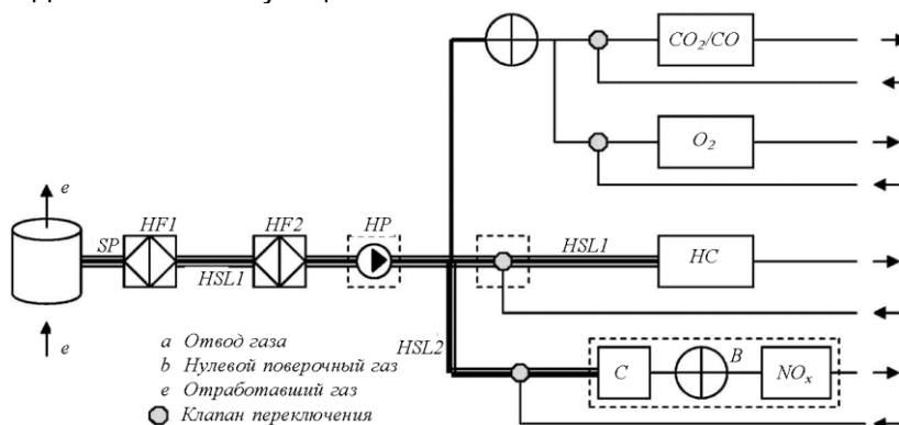
Рис. 1.1 Устройство системы анализа отработавших газов
