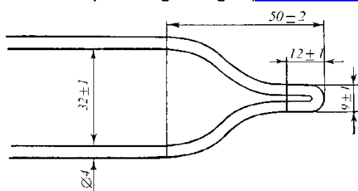
Fig. 1 Filament loop
