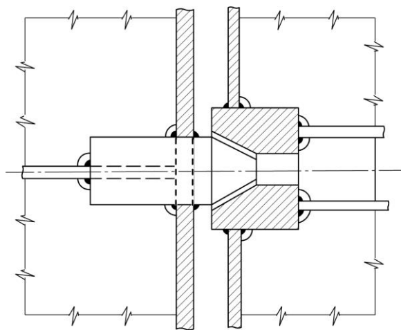
Рис. 7.4.2.8 Опора
