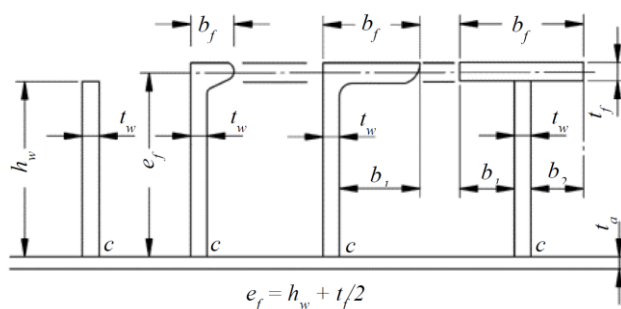
Рис. 7.10.6.31 Размеры ребра жесткости
