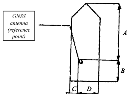
Fig. 5.3.1 Antenna position parameters:
