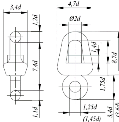
Fig. 7.1.3-7 Swivel
