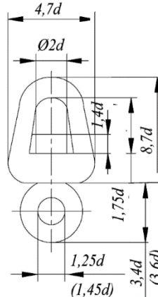
Fig. 7.1.3-7 Swivel
