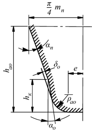
Fig. 4.2.2.7.3.2-3 Protuberance hob
