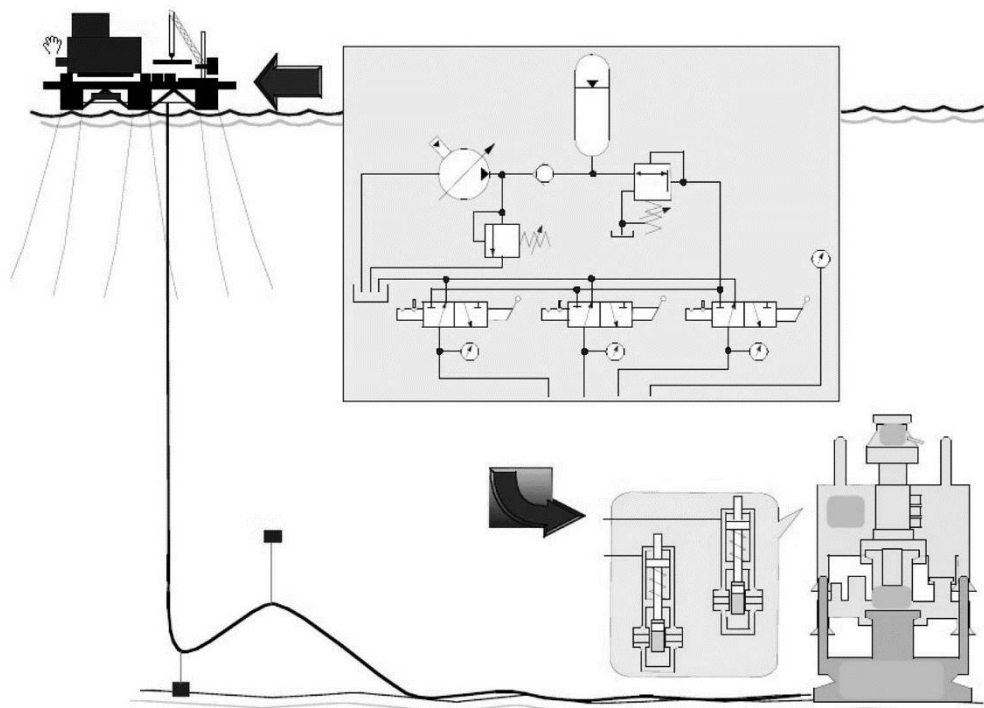
Рис. 2 Гидравлические системы с непосредственным гидроприводом
