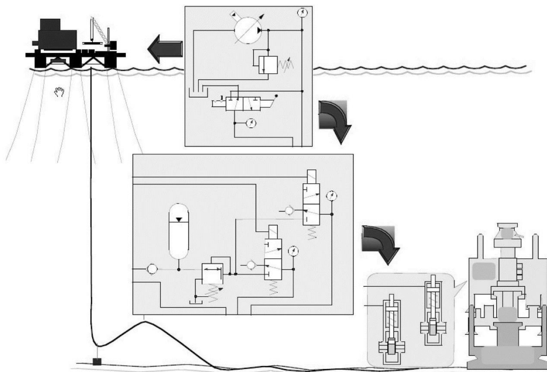
Рис. 5 Электрогидравлические системы с непосредственным приводом
