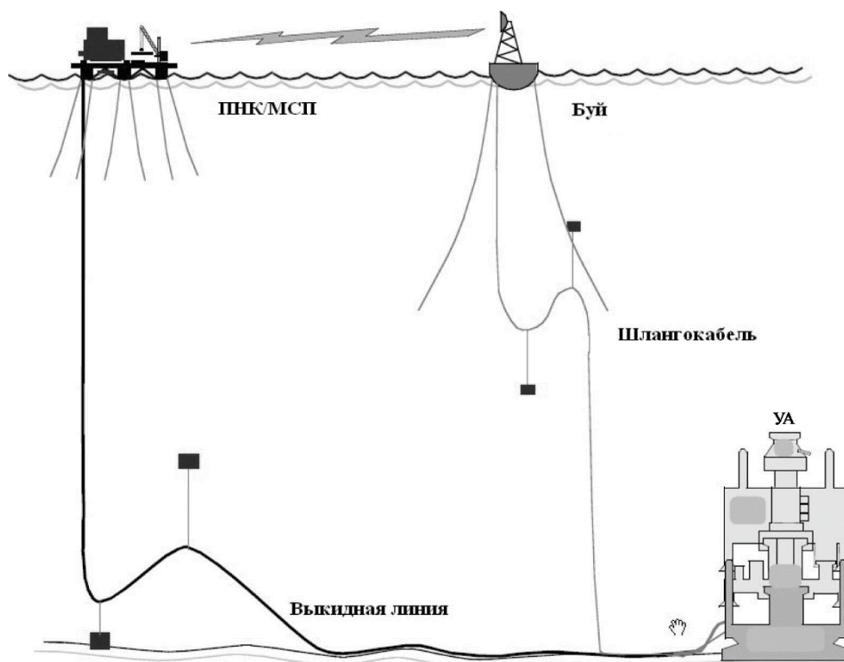
Рис. 8 Интегрированные буи контроля и управления (ICB)
