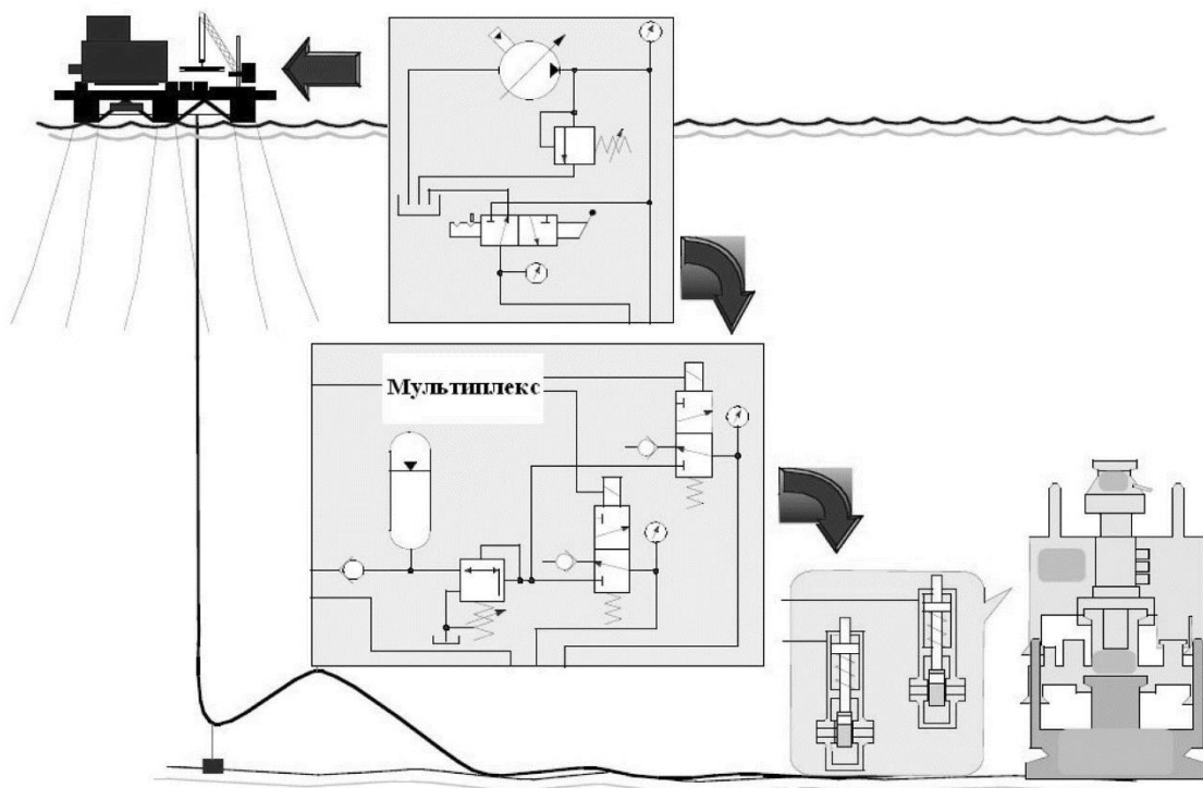
Рис. 6 Мультиплексные системы
