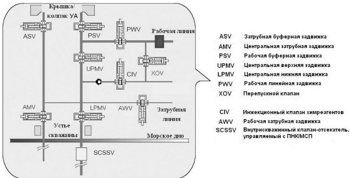
Рис. 1 Типовой комплект оборудования и арматуры
