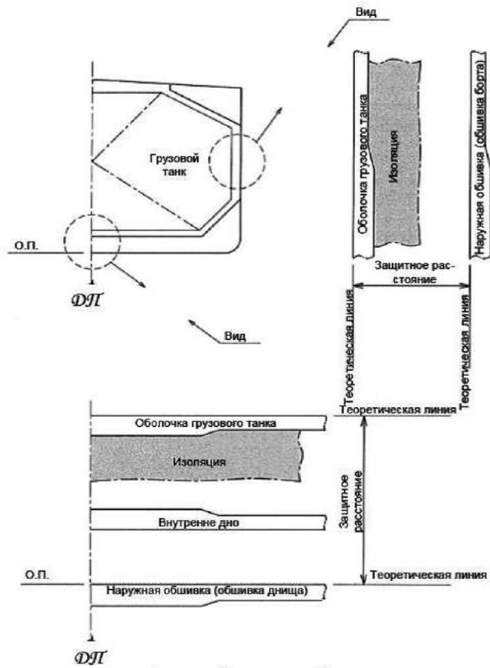
Рис. 2.5-1 Защитное расстояние для автономной призматической грузовой емкости
