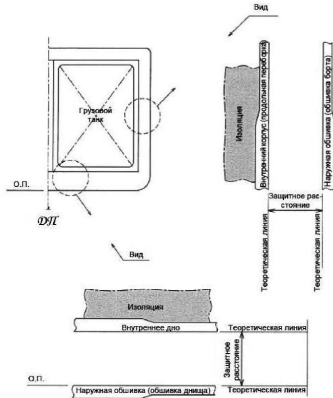
Рис. 2.5-2 Защитное расстояние для полумембранной грузовой емкости
