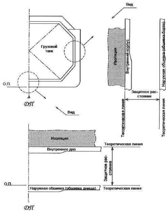
Рис. 2.5-3 Защитное расстояние для мембранной грузовой емкости
