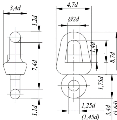
Fig. 7.1.3-7 Swivel
